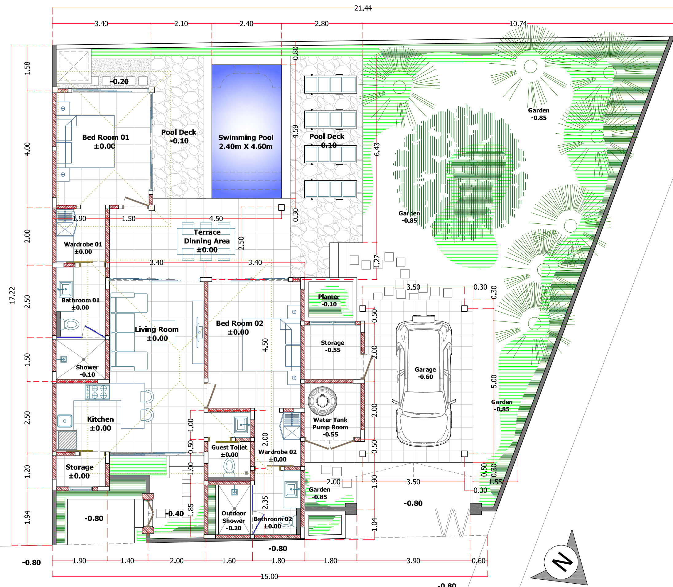
P L A N skala 1 : 80
